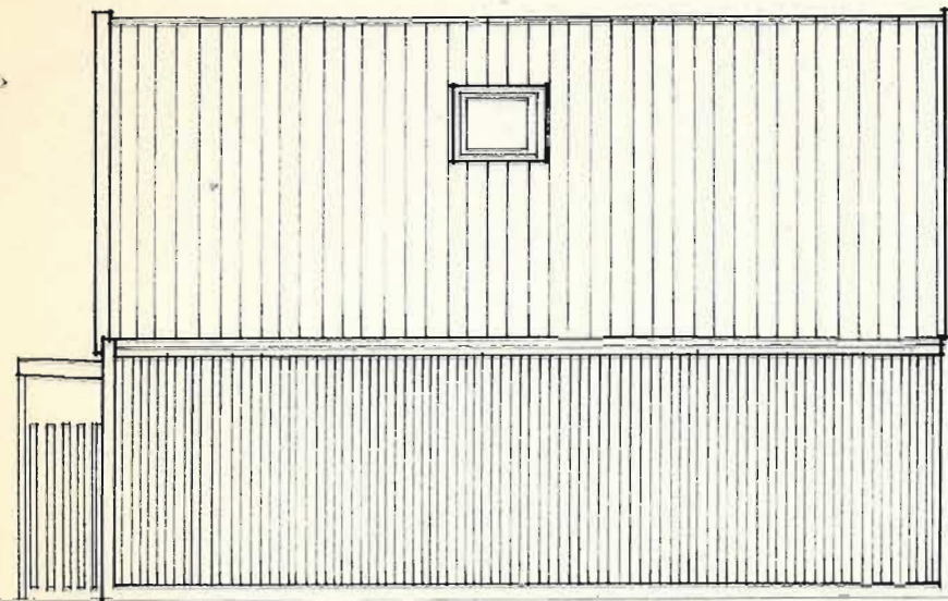
FASAD MOT TOMTGRÄNS EL MOTSV.
