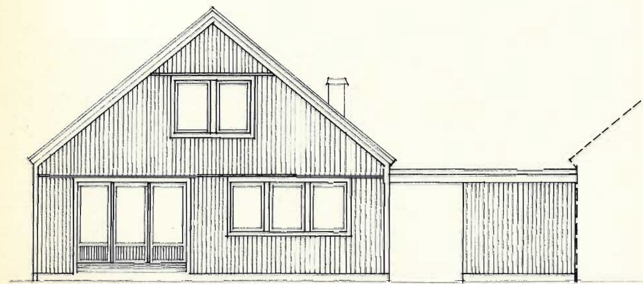
TRÄDGÅRDSFASAD
