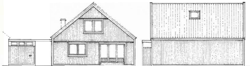
GATUFASAD
